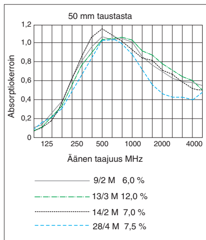
Äänen absorptiokertoimet ISO 354-standardin mukaan
